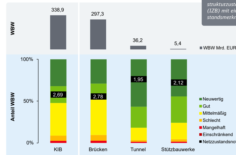
Abbildung 8: Mittlere Zustandsnote und Notenverteilung nach Wiederbeschaffungswert im Konstruktiven Ingenieurbau
